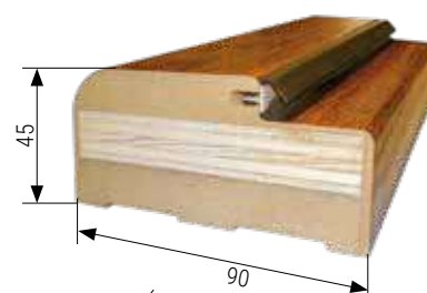
Ościeżnica stała wzmocniona OW-01
